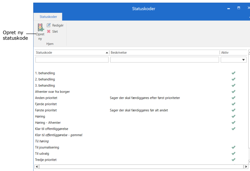
Figur 2: Vinduet "Statuskoder"
