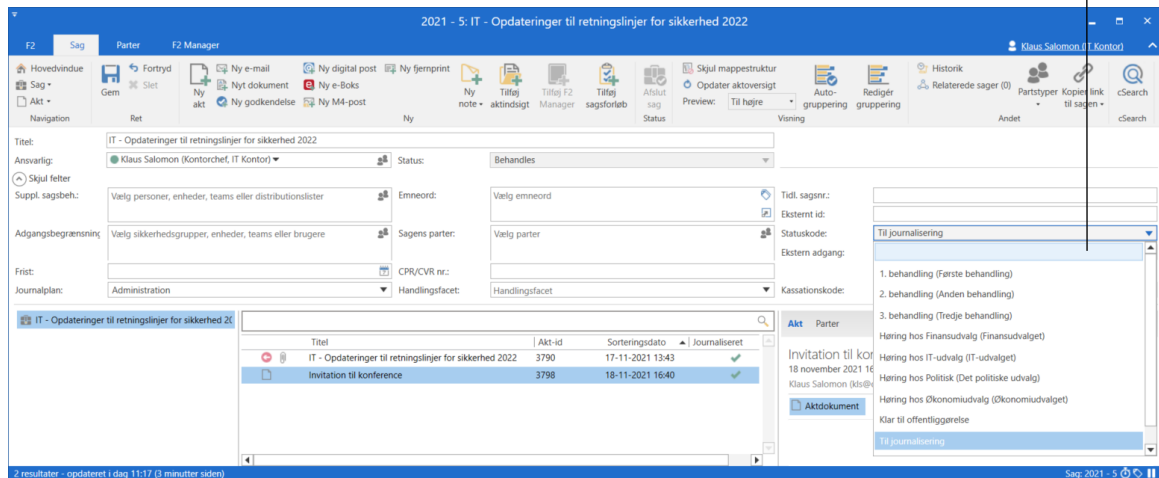
Figur 9: Fjern statuskode
